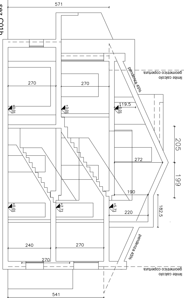
PIANO SOTTOTETTO
